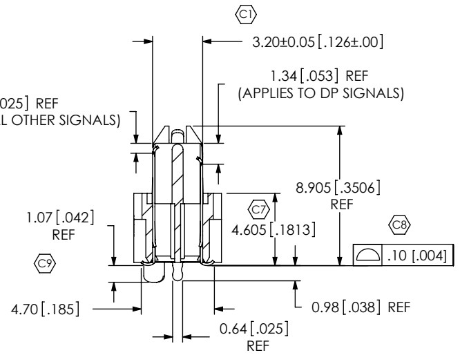
DETAIL 'B' SCALE 6 : 1 SE SIDE
