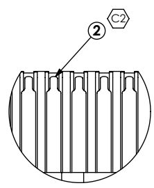
DETAIL 'B' SCALE 6 : 1 SE SIDE
