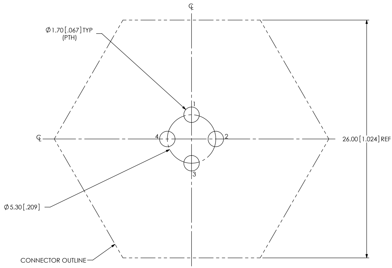
FIG 5 ACRK-16-03-X-T-BT-X-X SHOWN
