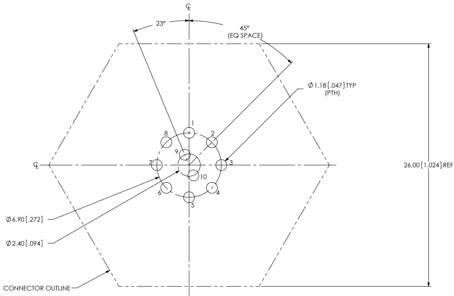
FIG 3 ACRK-16-02-X-T-BT-X-X SHOWN
