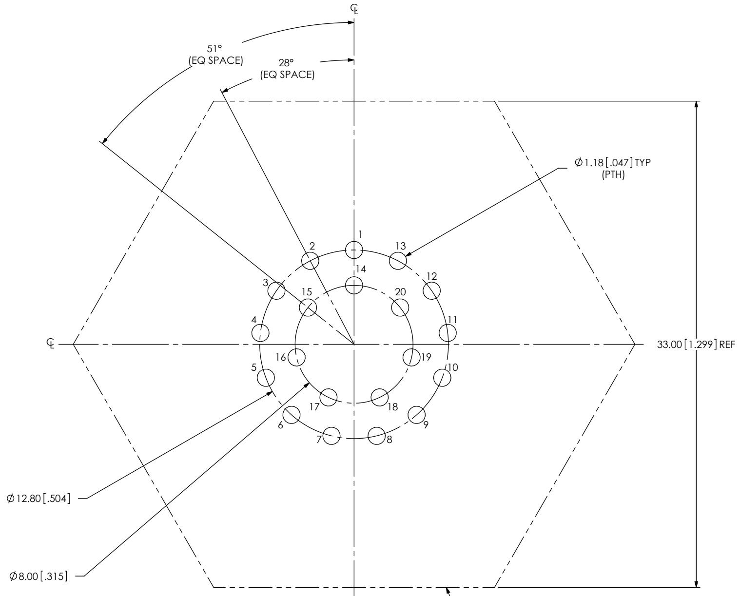
FIG 4 ACRK-22-02-X-S-BT-X-X SHOWN
