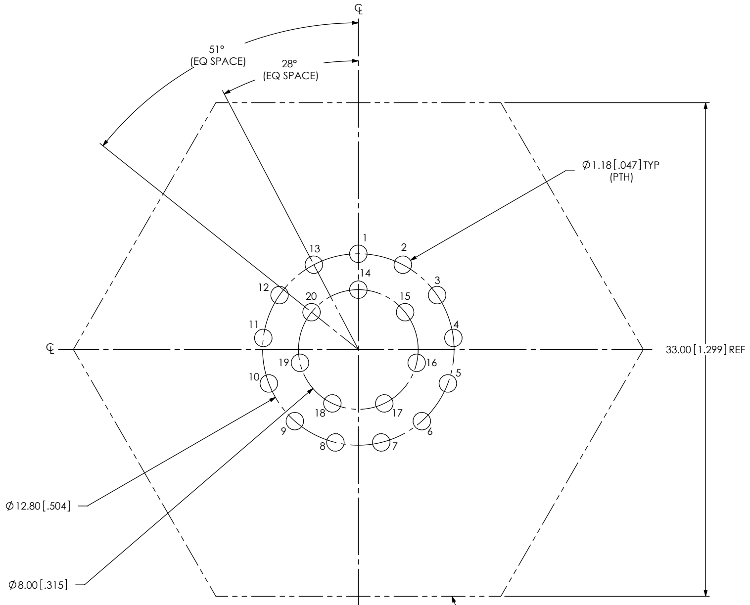
FIG 3 ACRK-22-02-X-T-BT-X-X SHOWN
