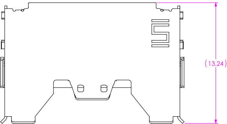
FIG 2 ARF6-16-X-RA SHOWN
