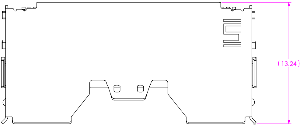
FIG 3 ARF6-24-X-RA SHOWN
