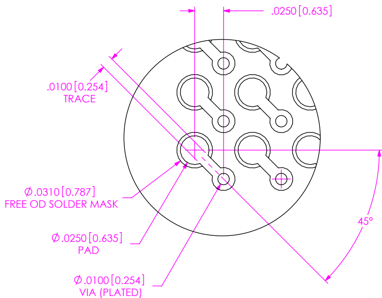
DETAIL 'B' SCALE 12:1
