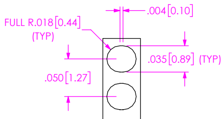
DETAIL 'B' SCALE 8 : 1
