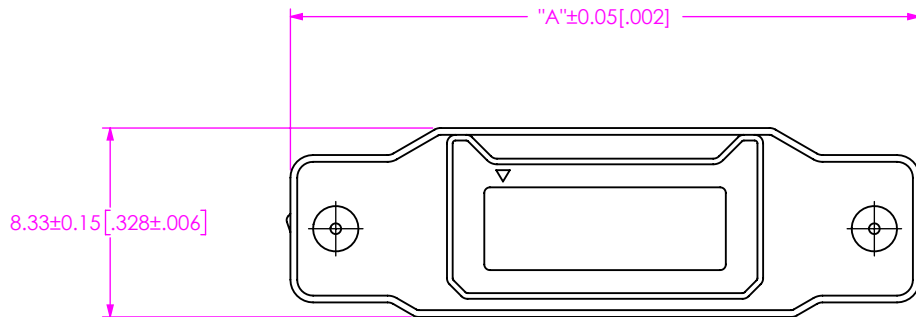
FIG 1 B1SDS-10-N-CS SHOWN
