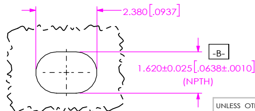
DETAIL 'B' SCALE 7 : 1
