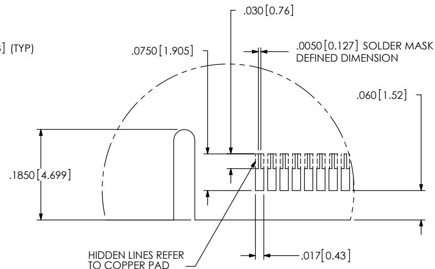
DETAIL 'B' SCALE 5:1
