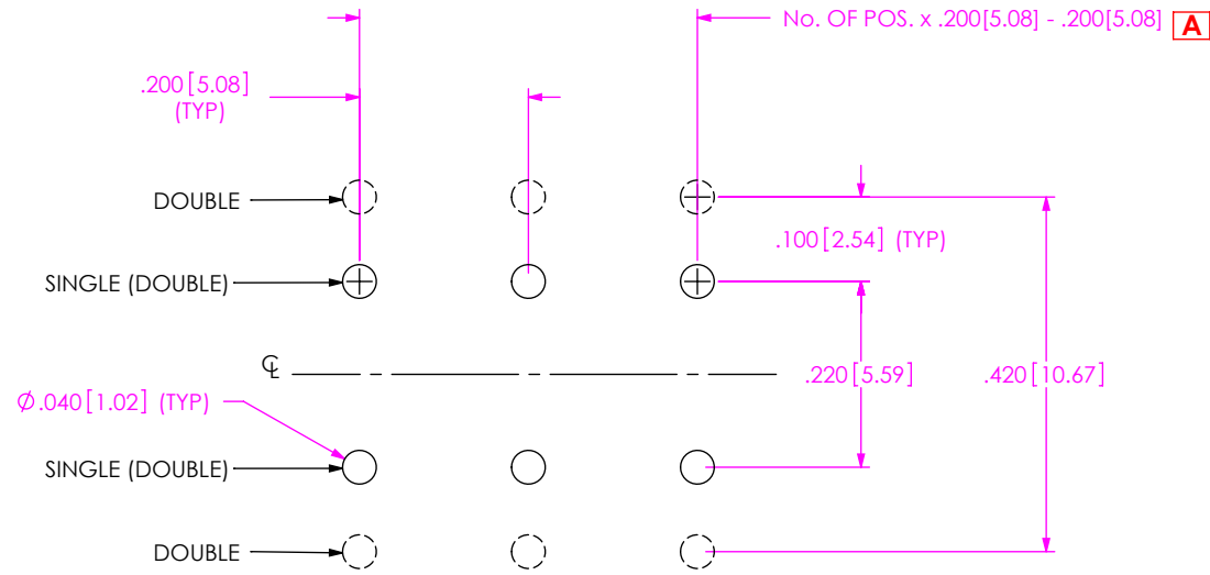
FIG.4 BTSW-2XX-02-X-X-XX-XXX SHOWN
