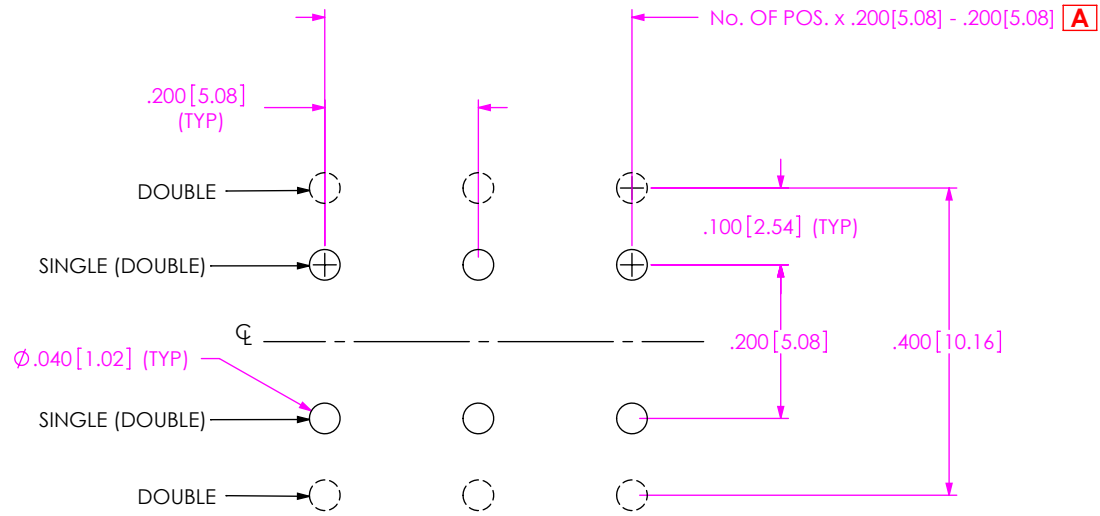
FIG.3 BTSW-2XX-01-X-X-XX-XXX SHOWN
