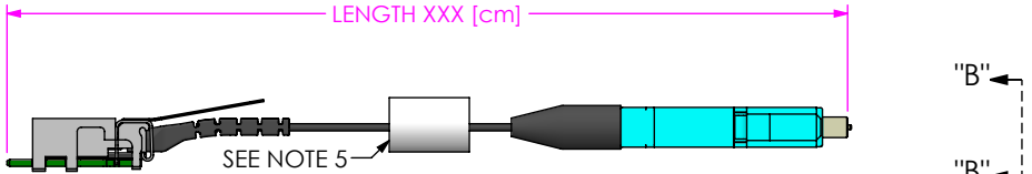
ETUO-X12-XX-XXX-0-1-1-5-07 SHOWN
