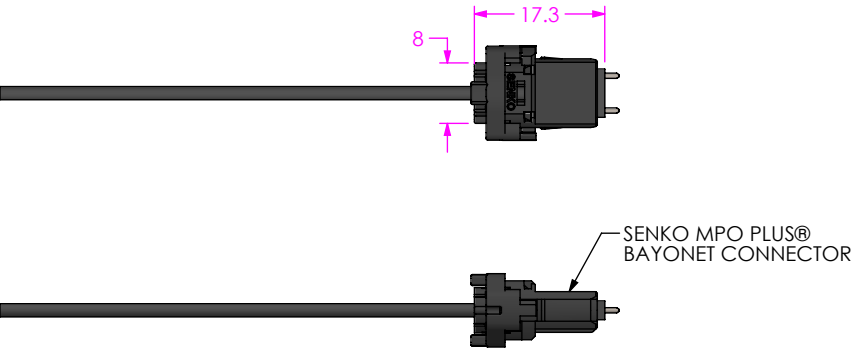
-7/-8 FIBER TYPE -0E END OPTION
