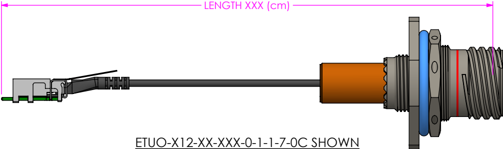
ETUO-X12-XX-XXX-0-1-1-7-0C SHOWN
