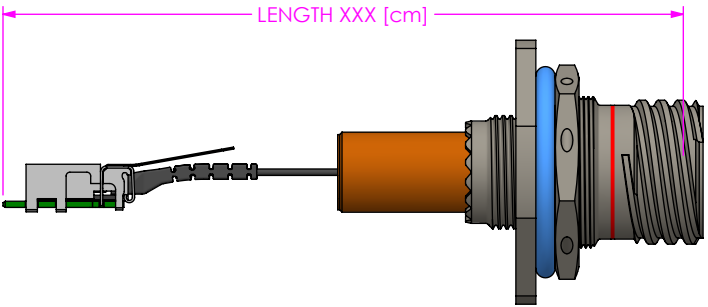
ETUO-X12-XX-XXX-0-1-1-5-0C SHOWN
