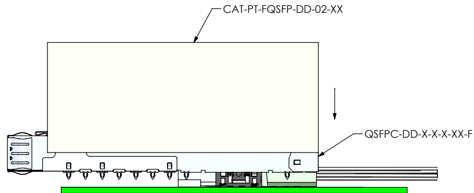
FIG 11 CAGE PRESS
