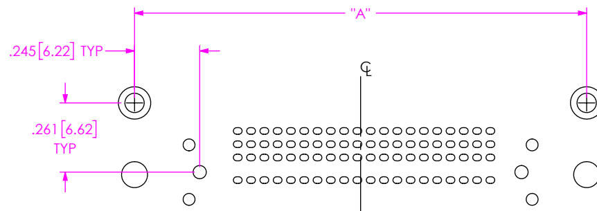
FIG 5 SEAM-XX-XX-X-XX-X-RA-XX-XX-FOOTPRINT (FOR GPXKM)
