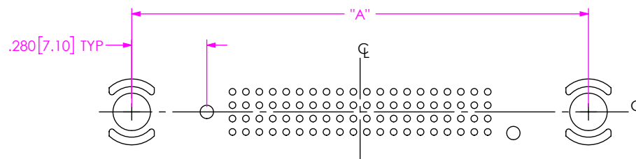
FIG 6 SEAF-XX-XX.X-XX-XX-X-XX-FOOTPRINT (FOR GPXKM)
