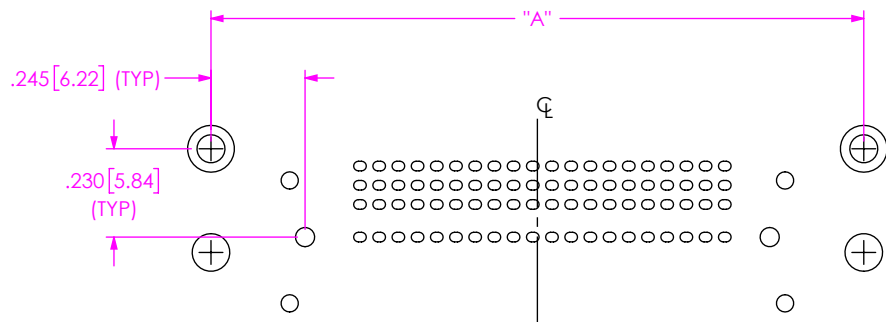
FIG 3 SEAF-XX-XX-X-XX-X-RA-XX-XX-FOOTPRINT (FOR GPXKM)
