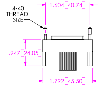
EDGE MOUNT
