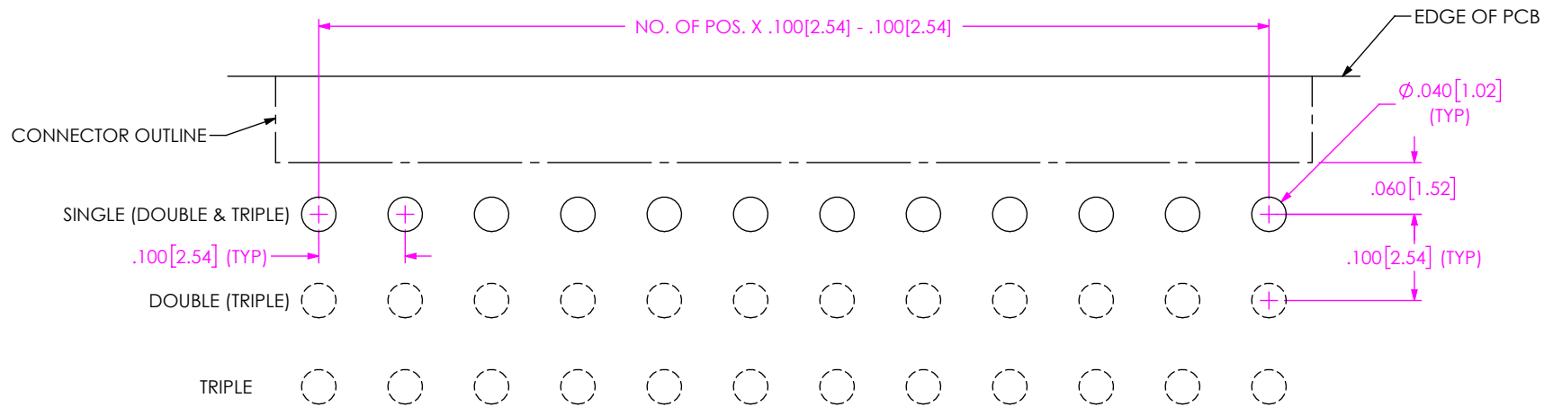
FIG 5 HTSW-1XX-XX-XXX-X-RA-FOOTPRINT SHOWN
