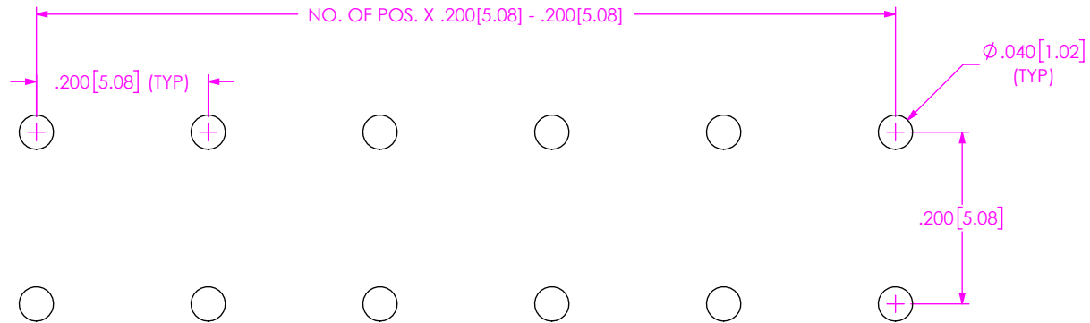
FIG 4 HTSW-2XX-XX-XXX-Q-FOOTPRINT SHOWN
