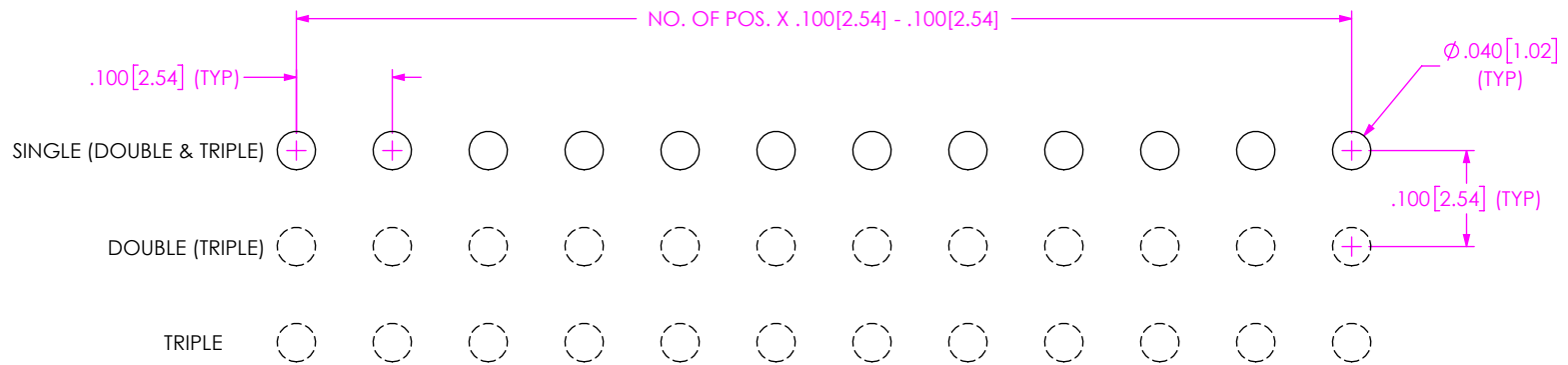
FIG 1 HTSW-1XX-XX-XXX-X-FOOTPRINT SHOWN
