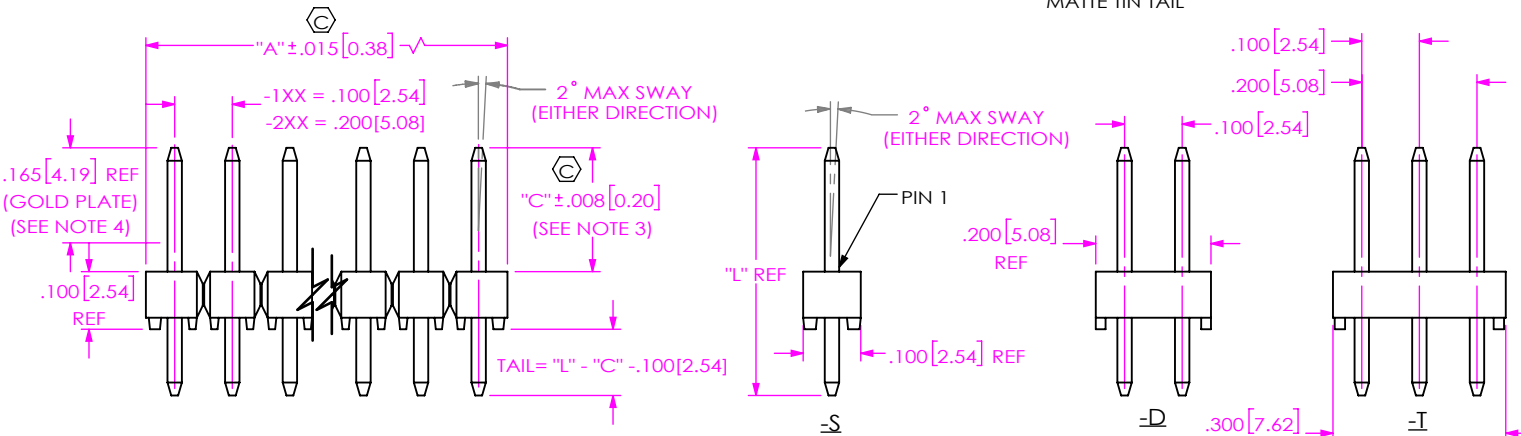
FIG 1 MTSW-XXX-XX-X-X-XXXX SHOWN
