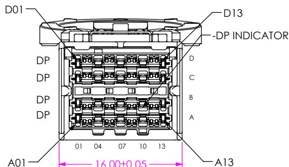
FIG 1 NVACE-DP-XX-4-X-X-A-X-1 SHOWN
