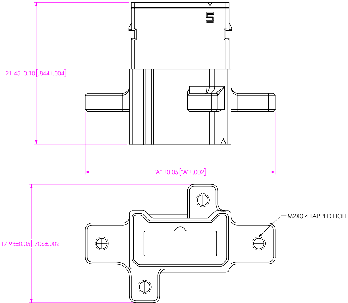
FIG 1 P1PDS-10-N SHOWN
