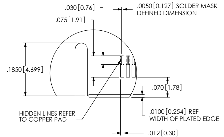
DETAIL 'B' SCALE 5:1
