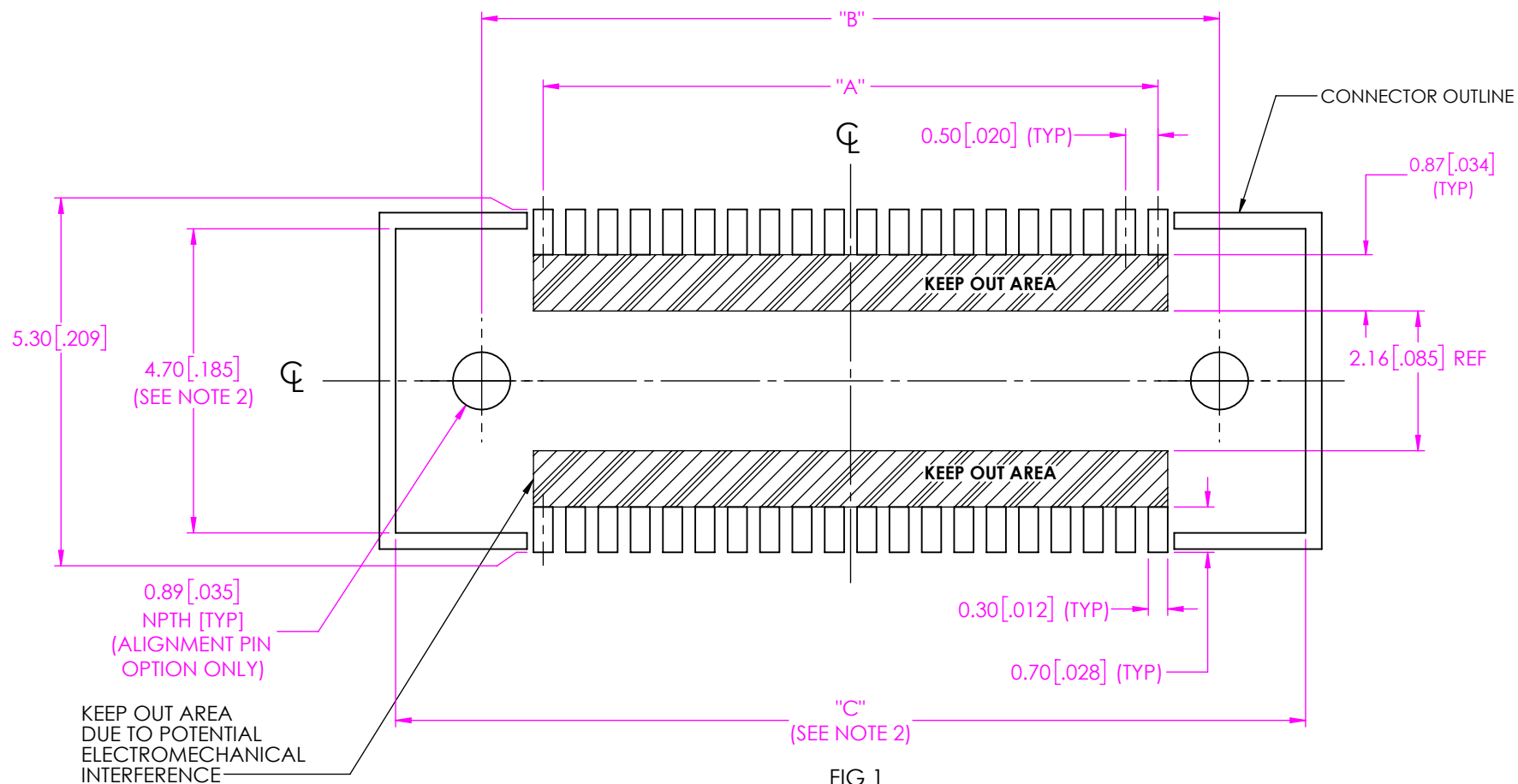
FIG 1 SLH-020-X.XX-X-D-A SHOWN
