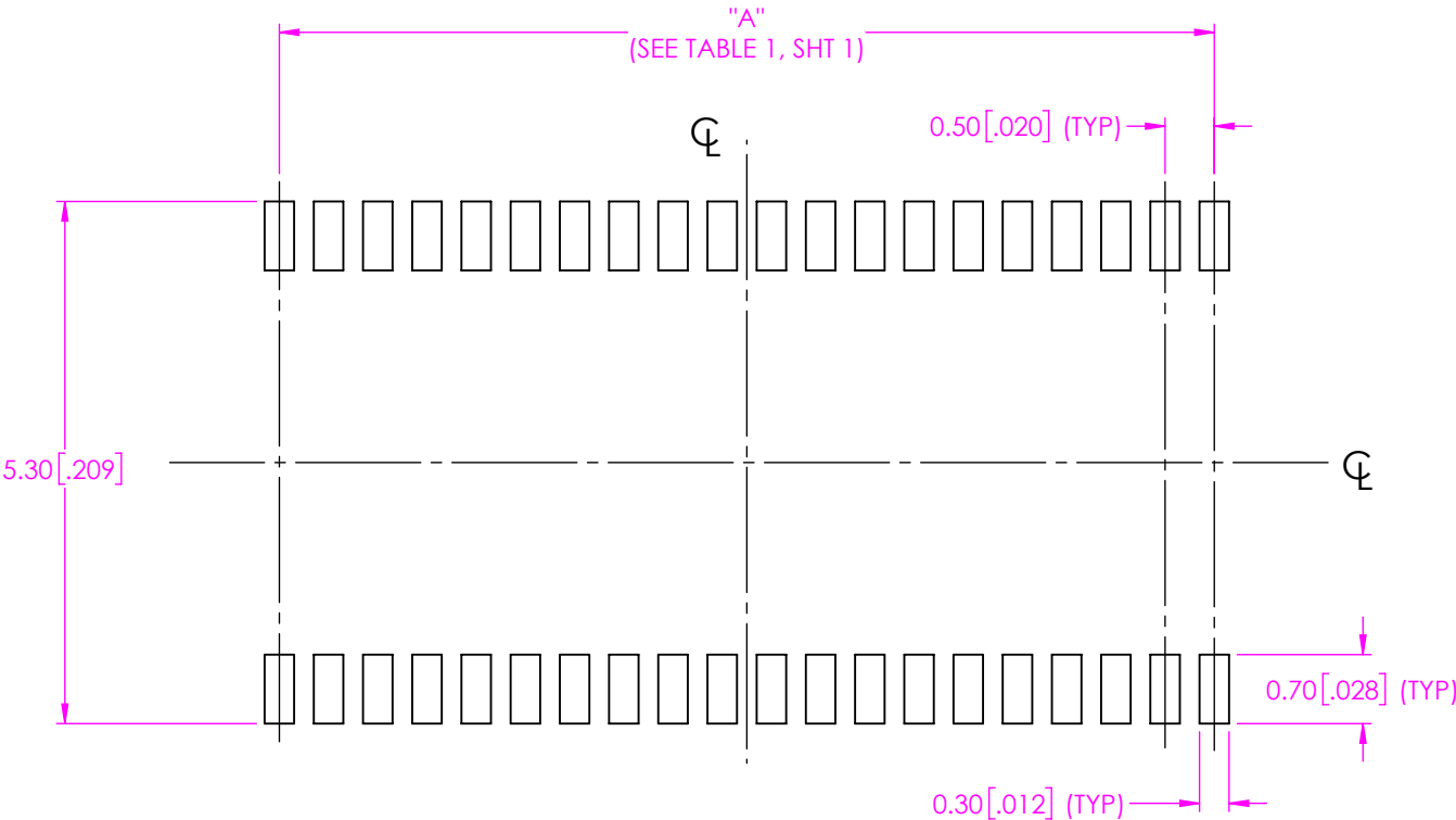
FIG 2 SLH-020-X.XX-X-D-A SHOWN
