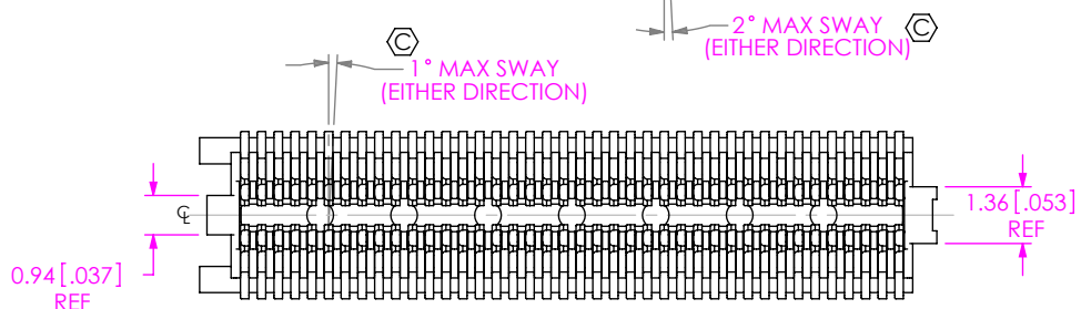
FIG 1 ST4-40-1.00-X-D SHOWN
