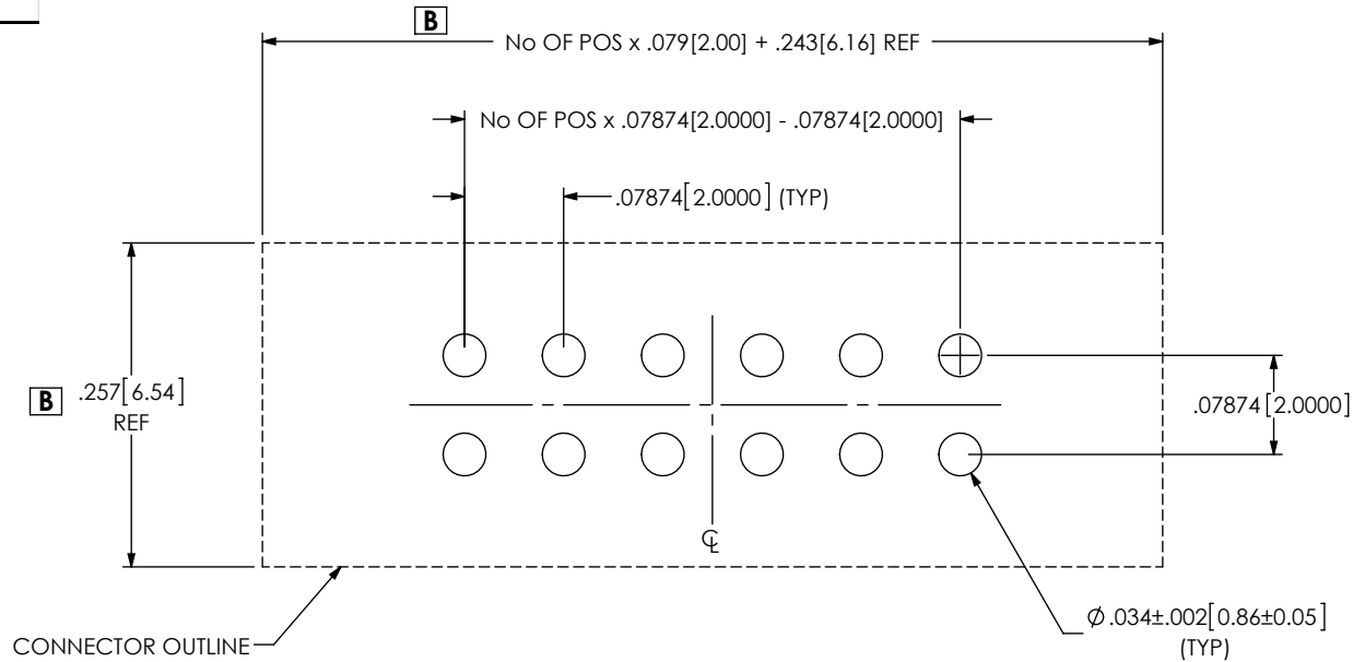
B FIG 1 STMM-1XX-XX-XX-D SHOWN
