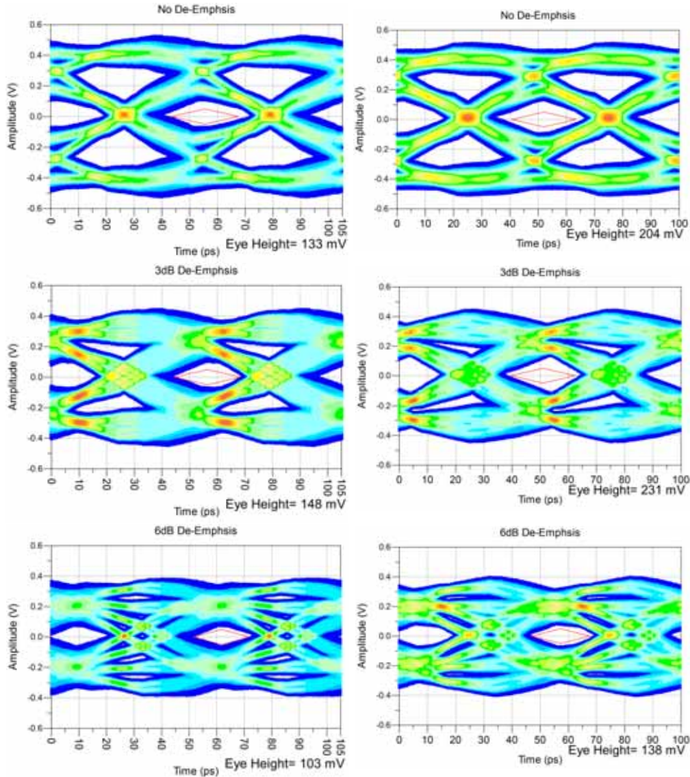
Long Row Output Eye : 19Gbps
